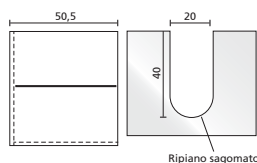
Ripiano sagomato
