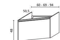
Base lavatrice
