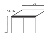
Base lavatrice
