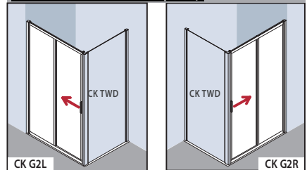
Угол: CK G2R/L и CK TWD (страница 16)
