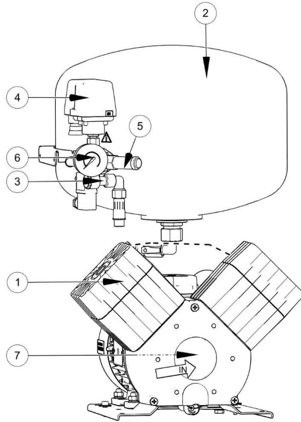
Fig. 1: Compressor without dryer DK50 2V MOBILE MINI 409202005-302
