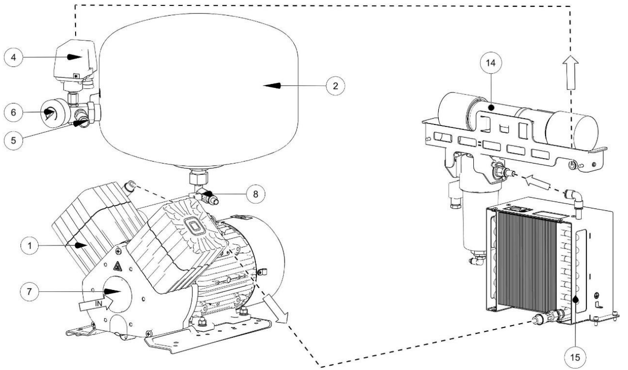
Fig. 2: Compressor with dryer DK50 2V/M MOBILE MINI 4092020A5-305 / 4092020A5-307
