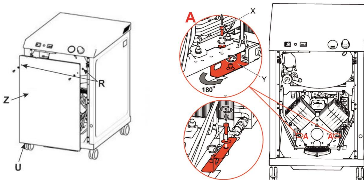
Obr. 4: Odfixovanie agregátu
