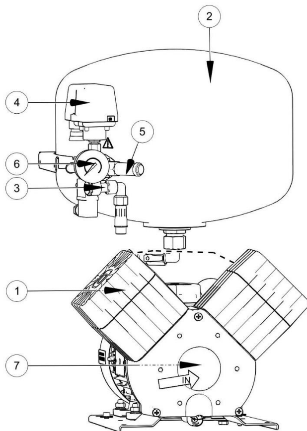
Obr. 1: Kompresor bez sušiča DK50 2V MOBILE MINI 4092020 05-302
