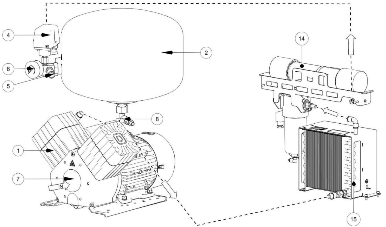
Abb.2: Kompressor mit Trockner DK50 2V/M MOBILE MINI 4092020A5-305 / 4092020A5-307
