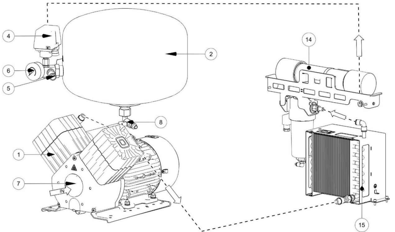
Obr. 2: Kompresor so sušičom DK50 2V/M MOBIE MINI 4092020A5-305 / 4092020A5-307
