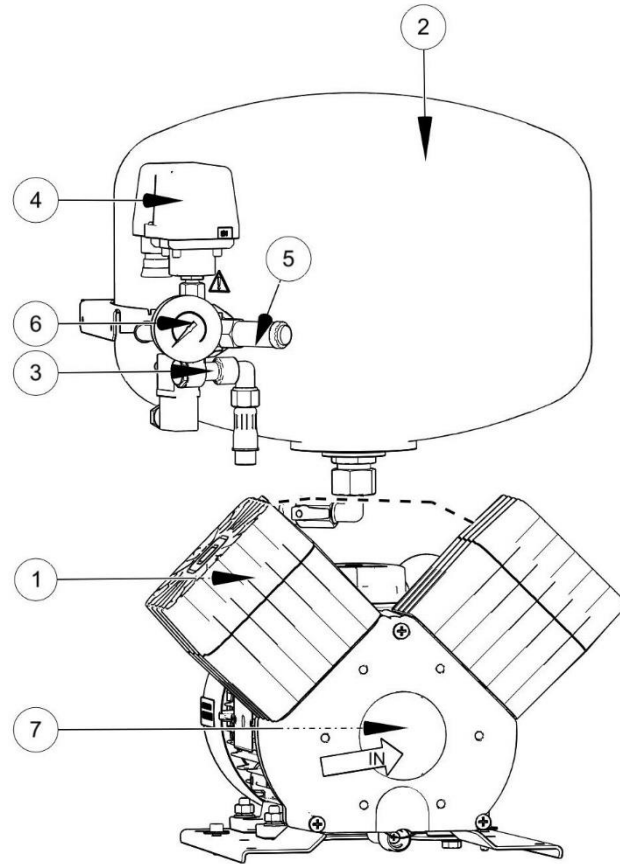
Abb. 1: Kompressor ohne Trockner DK50 2V MOBILE MINI 409202005-302
