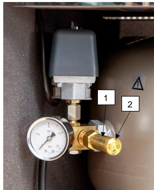
Obr. 7: Kontrola poistného ventilu
