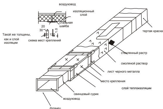
Изоляция путем оборачивания прямоугольного воздуховода листовым материалом
