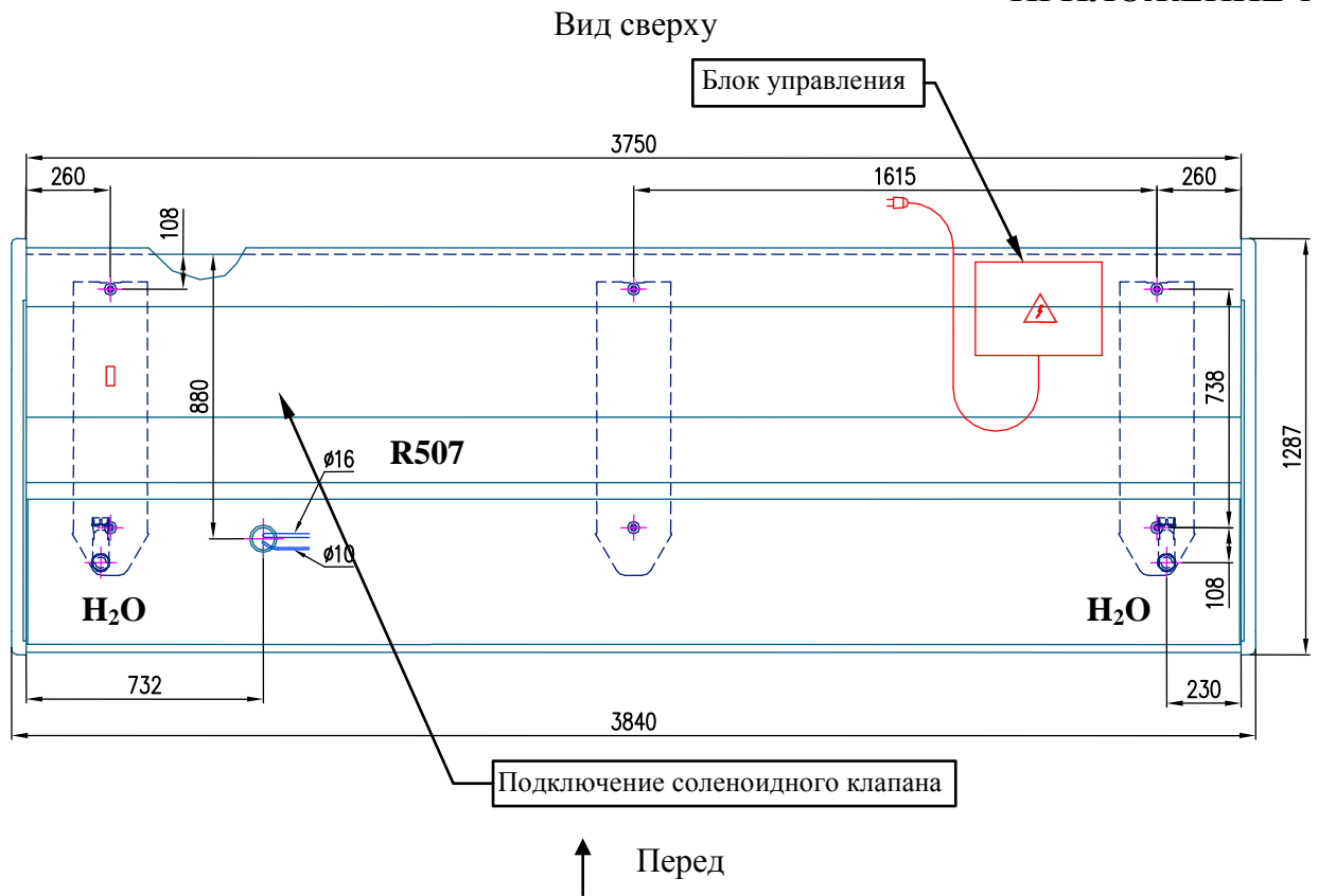
Рис. П1-4. «НЕМИГА EXTRA» 375
