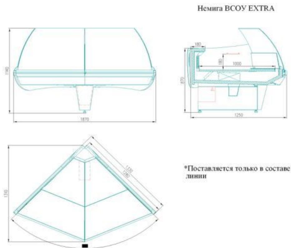
Рис. 1б. Схема витрины «НЕМИГА EXTRA» УН 90 ВС
