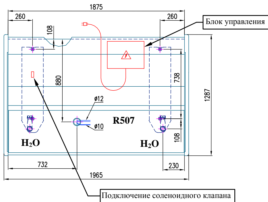
Рис. П1-2. «НЕМИГА EXTRA» 187
