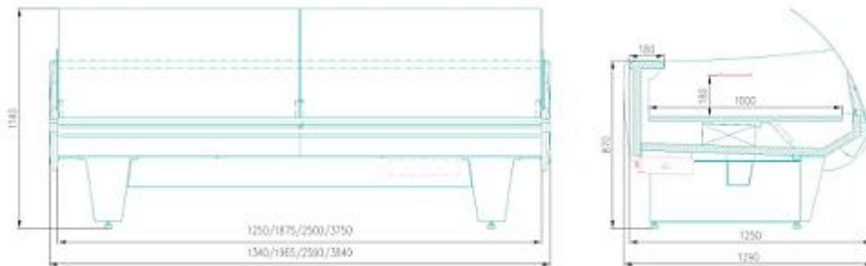
Рис. 1а. Схема витрины «НЕМИГА EXTRA» BC, BCn
