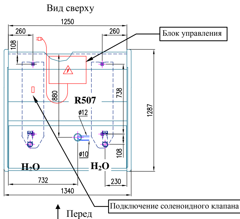
Рис. П1-1. « НЕМИГА EXTRA » 125
