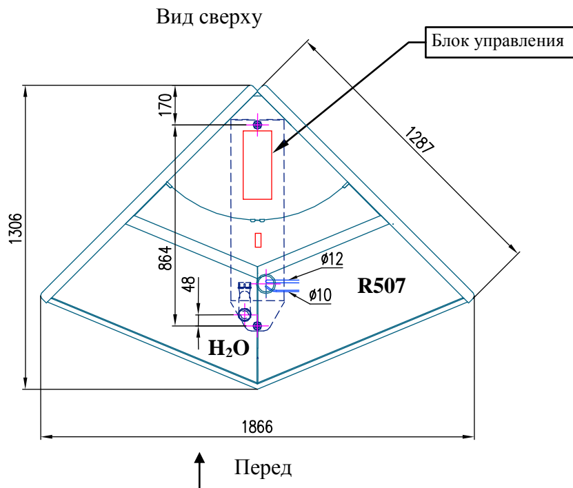
Рис. П1-5. «НЕМИГА EXTRA» УН 90
