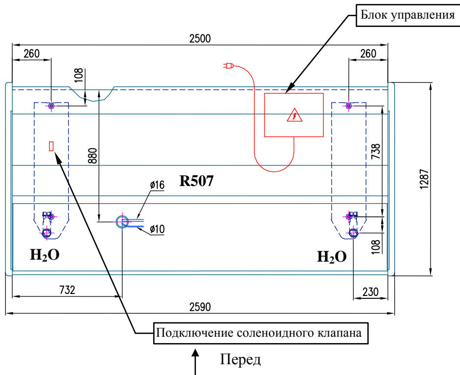
Рис. П1-3. «НЕМИГА EXTRA» 250
