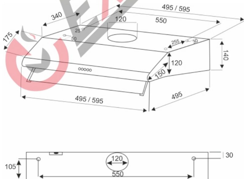
Рис. 1 Внешний вид кухонной вытяжки и схема размеров
