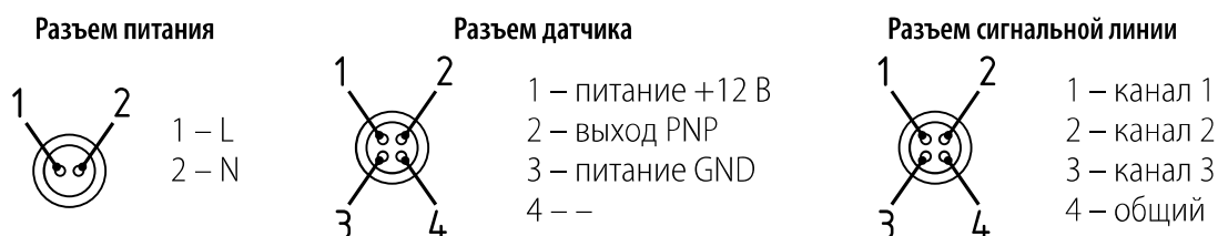
Рисунок 2. Распайка внешних разъемов сигнализатора.
