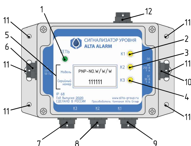
Рисунок 1. Внешний вид, органы индикации и разъемы сигнализатора.
