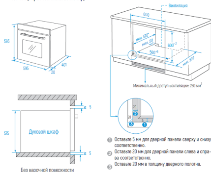
Схема (Горизонтальный шкаф)
