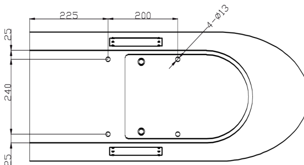
ВИД СНИЗУ
