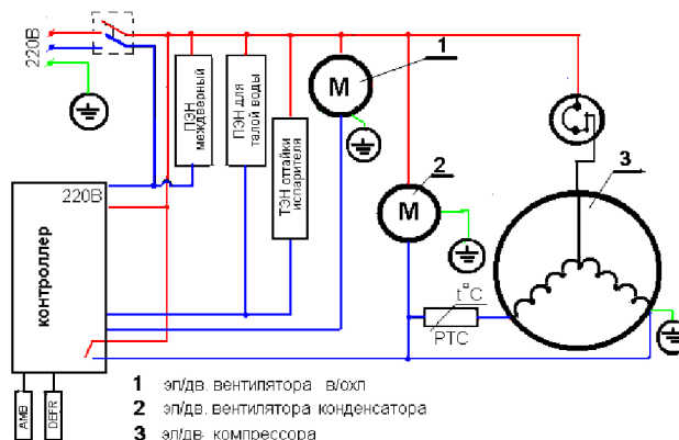
17.2 Электрическая схема стола ВТ.
