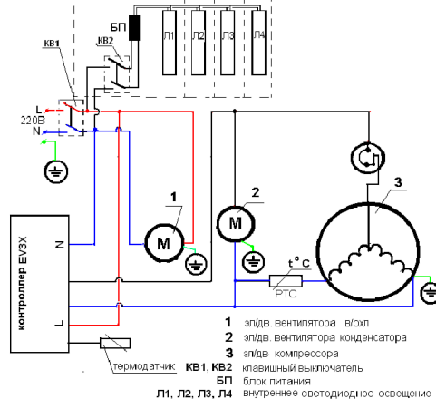
17.2 Электрическая схема стола ВТ.
