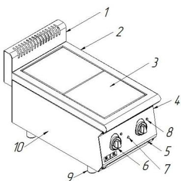
Плита электрическая ПЭ-2-121-МХ
