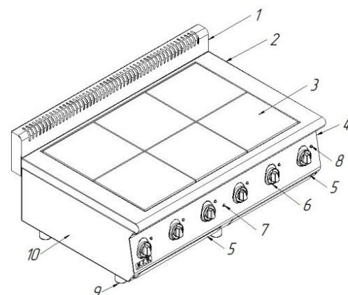
Плита электрическая ПЭ-6-121-МХ
