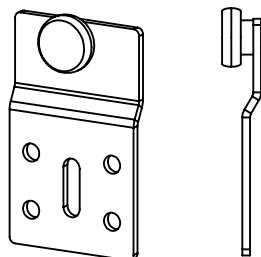
21. Ролик 2 - 2 шт
