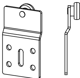
20. Ролик 1 - 2 шт
