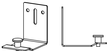
22. Ролик 3 - 2 шт
