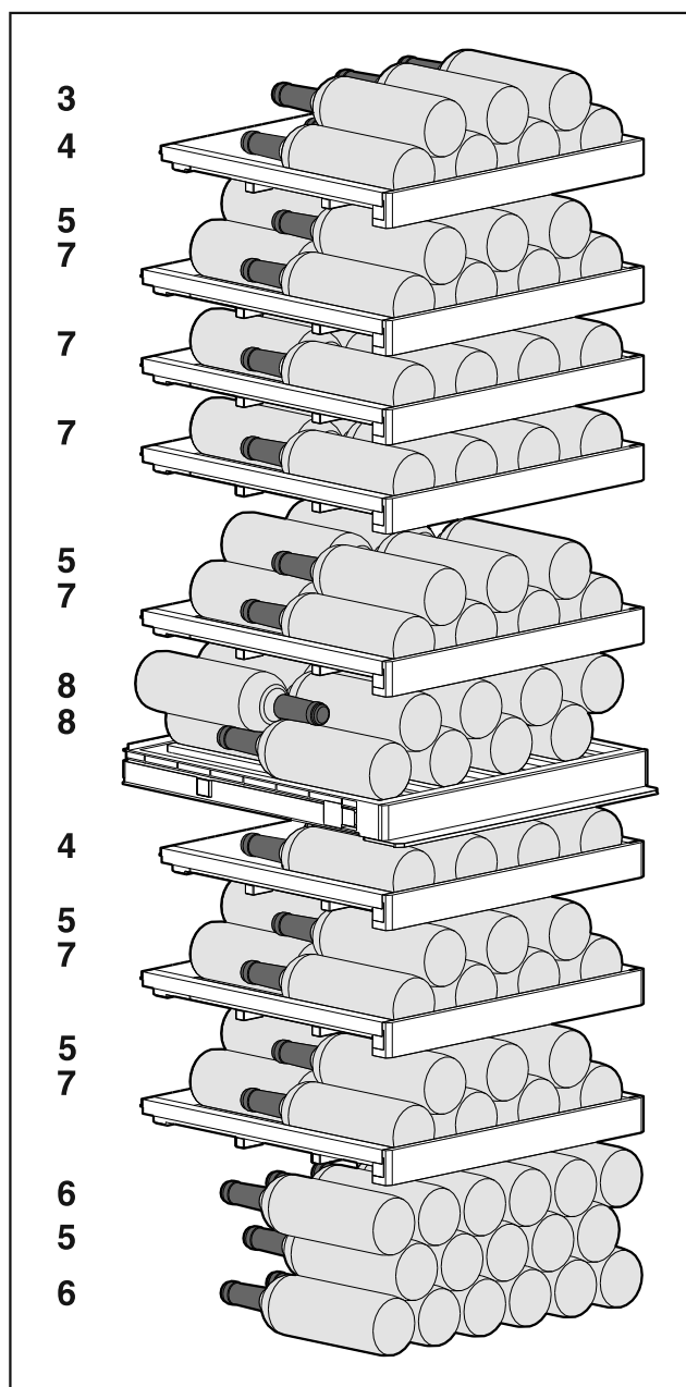
Fig. 12 Всего 106 бутылок (для бордоских винных бутылок 0,75 л)
