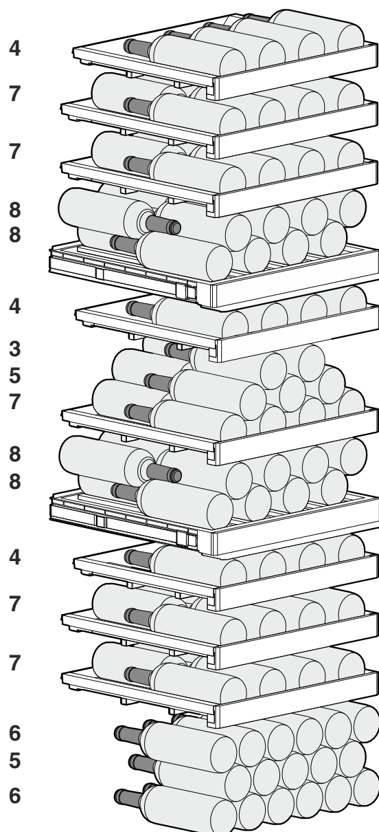
Fig. 13 Всего 104 бутылки (для бордоских винных бутылок 0,75 л)
