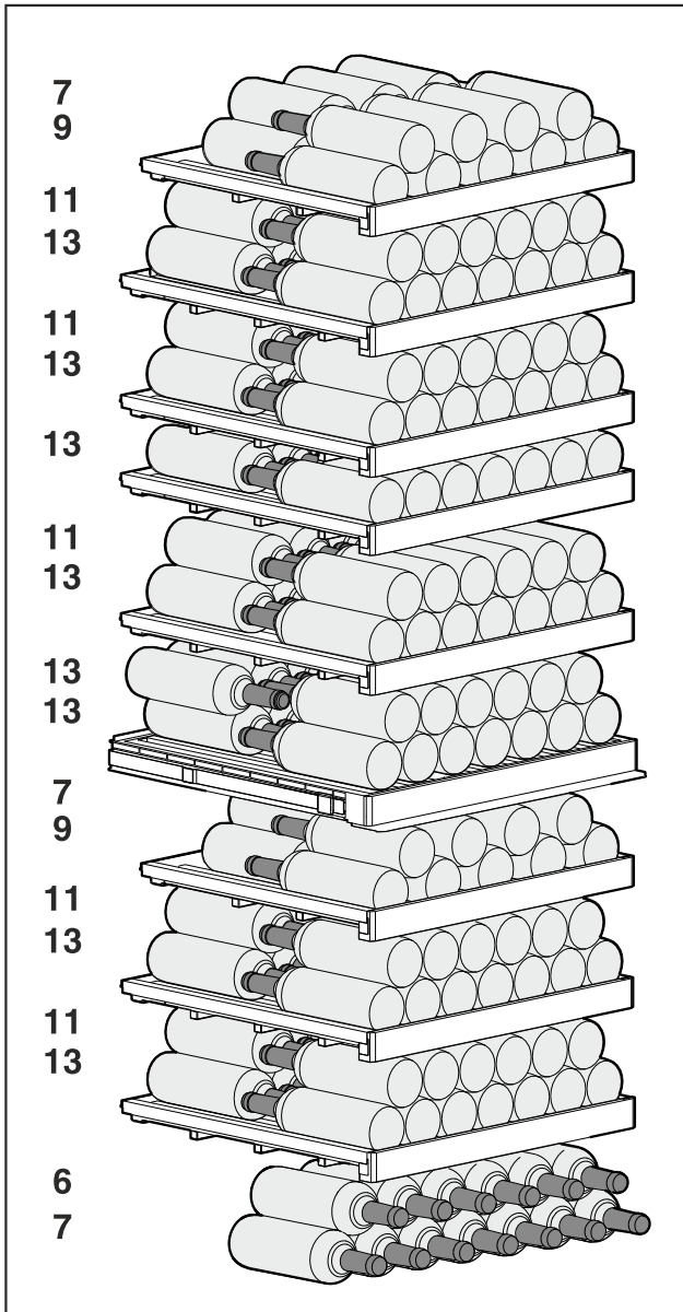
Fig. 16 Всего 204 бутылки (для бордоских винных бутылок 0,75 л)
