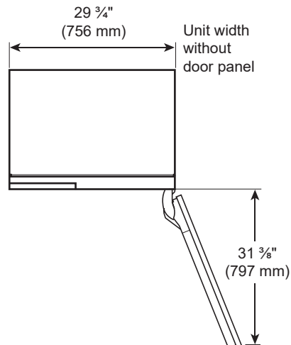
DOOR OPEN 115°
