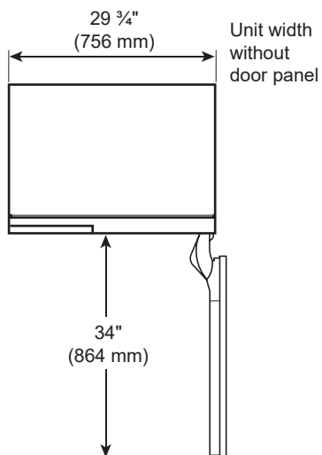
DOOR OPEN 90°
