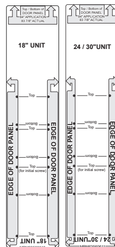
TOP / BOTTOM DOOR PANEL
