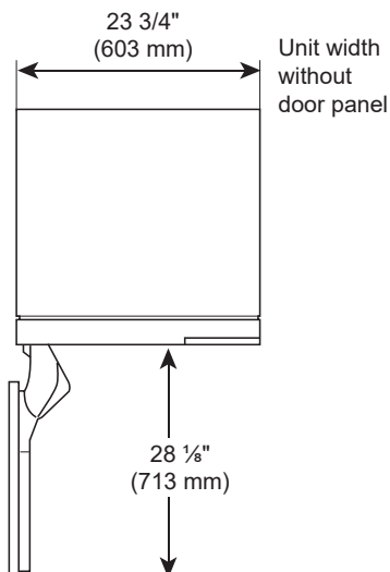
DOOR OPEN 90°
