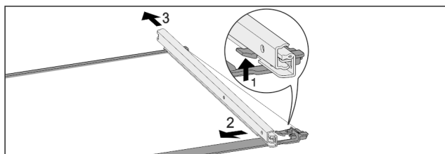
Fig. 124 Стеклянная пластина с направляющими
